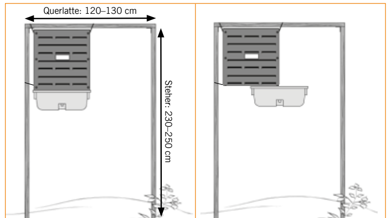
Einfallensteher selber bauen: Lattenstärke: 5 x 5 cm | Querlatte: 120–130 cm | 2x Steher: 230–250 cm
